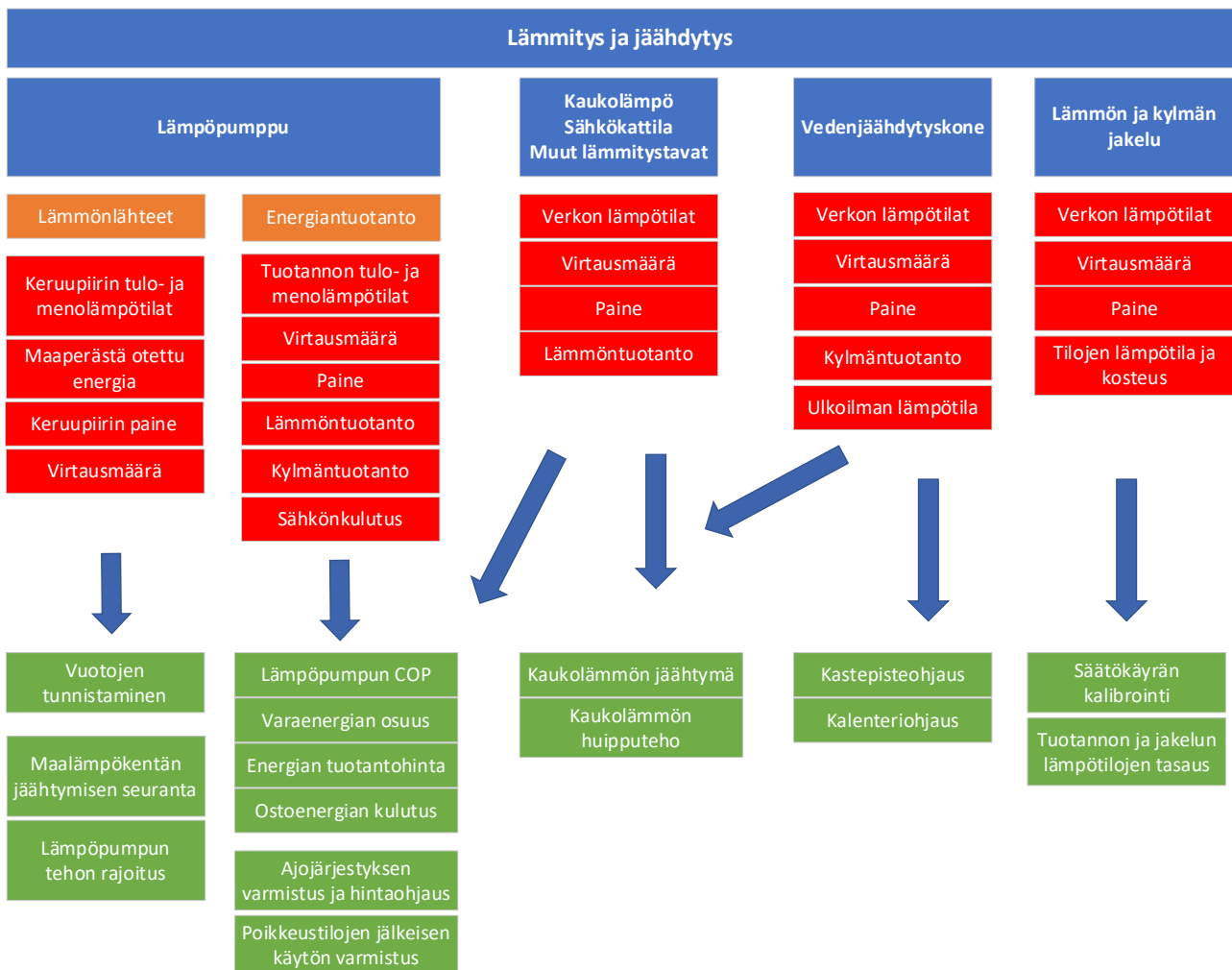
Kuva 4. Hybridienergiajärjestelmän mittauksia ja menettelyjä.
