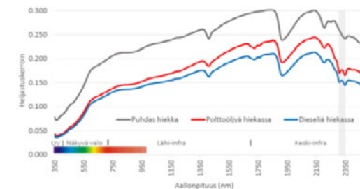
Polttoöljy ja diesel aiheuttavat kaksi vierekkäistä absorptiopiirrettä 2311-2351 nanometrin (nm) välillä. Projektissa tutkitaan, kuinka pieniä hiilivetypitoisuuksia näkyvän valon ja infrapuna-alueen spektroskopiolla voidaan tunnistaa.
